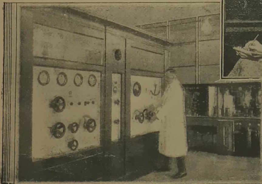
Aparato emisor: Válvula gobernadora (a la izquierda); las seis válvulas principales; las tres válvulas de modulación (a la derecha)
