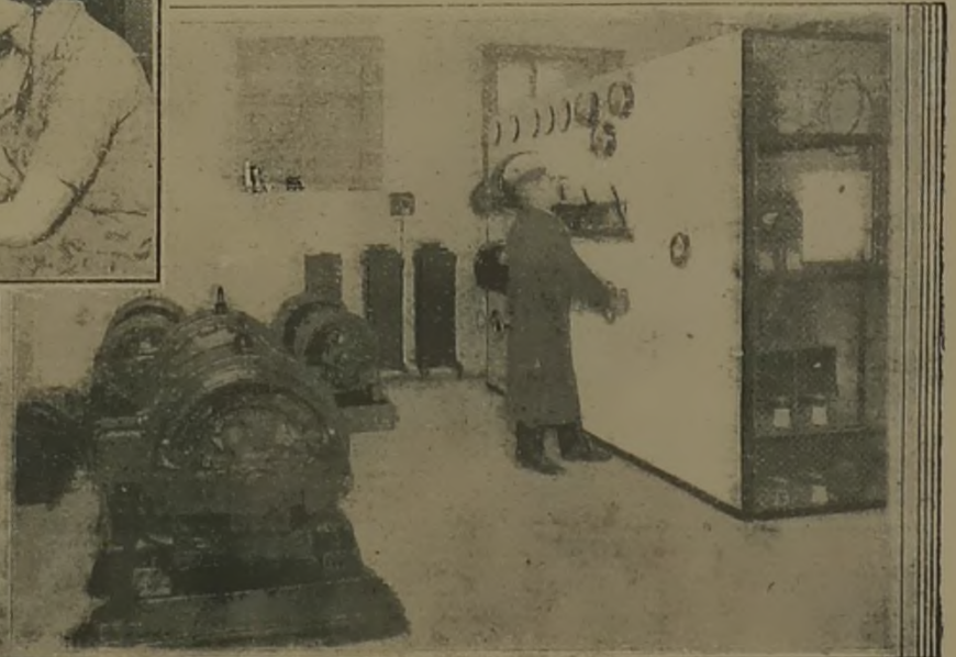
Los grupos transformadores de corriente continua en alterna con su cuadro de distribución
