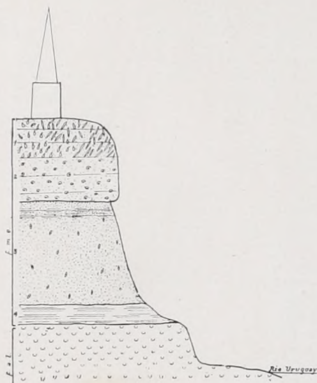
Fig. 2. — Perfil transversal esquemático de la barranca de Punta Gorda, donde se levanta la Pirámide erigida en homenaje a los descubridores del Río de la Plata; f, m, e , formación marina entre- rriana (1, depósitos arenoarcillosos con abundancia de valvas de ostras, predominando en algunos sitios ostras de valva angosta y alargada; 2, bancos calcáreos con moldes internos e impresiones externas de moluscos bivalvos y gasterópodos; 3, arena blanca fina disgregable, con alternancias de pequeños estratos de arcilla verde en la parte superior y valvas del braquiópodo Lingula ; 4, arcilla verdosa); f, a, l , formación araucana loessoide, de origen continental. Escala de alturas, 1:400.
