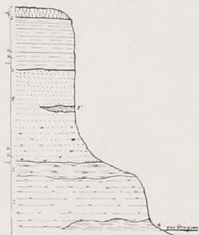
Fig. 1.—Perfil transversal esquemático de la barranca del río Uruguay, en la cabaña "El Recreo", 10 kms. al Sur de Carmelo.
