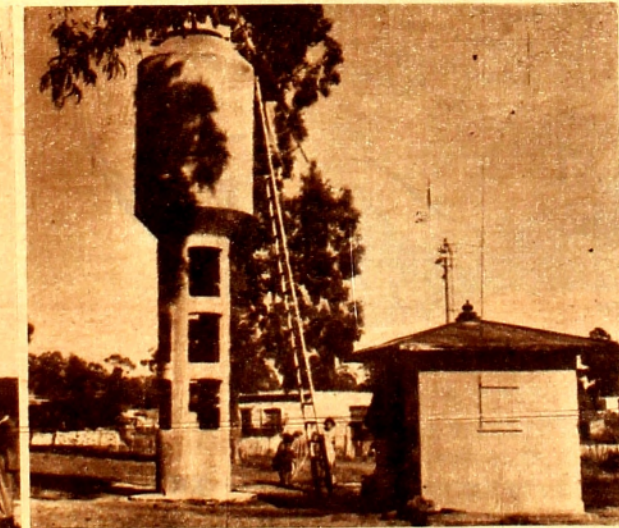
Moderno tanque para el suministro de agua potable a zonas que no cuentan con red de cañerías.
