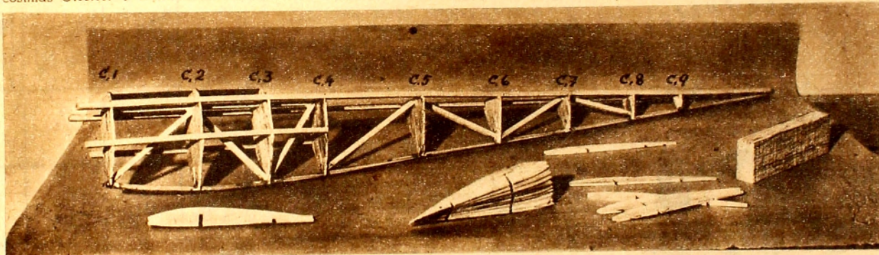
DETALLE DEL FUSELAJE DEL AVION, EN MADERA DE Balsa, Y EN UN PERIODO AVANZADO DE CONSTRUCCION, EN EL GRABADO SE APRECIAN PERFECTAMENTE LAS CUADERNAS: C-1, C-2, ETC., DE QUE SE HABLA EN EL TEXTO. LA LONGITUD TOTAL DEL FUSELAJE ES DE 1.040 MM. EL TARUGO DE MADERA QUE SE VE A LA DERECHA ES EL QUE SIRVE PARA LA CONSTRUCCION DE LA "NARIZ".
