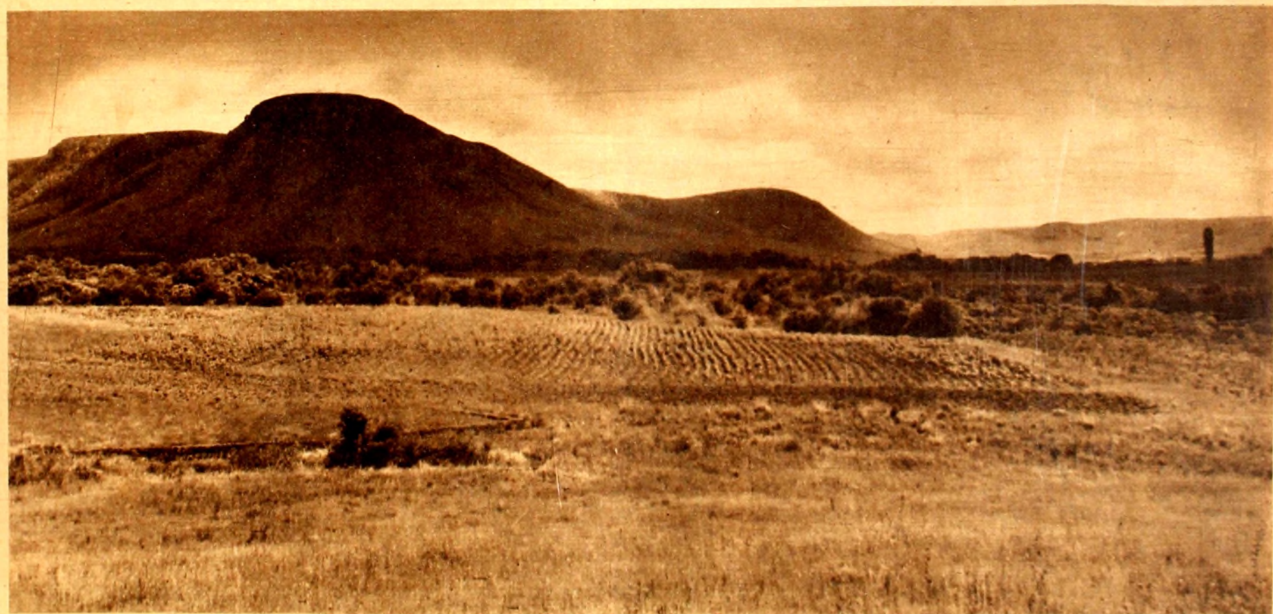
BORDE DE LA CUCHILLA NEGRA, TIPO DE CUCHILLA MESA PROTEGIDA POR UN MANTO BASALTICO. RIVERA.
