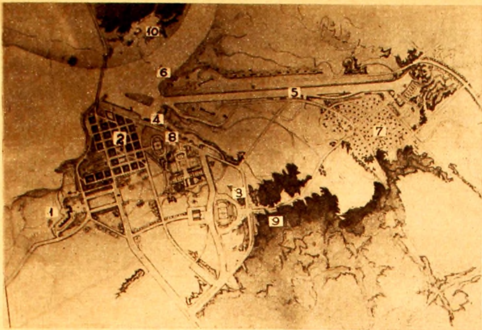
PROYECTO DE URBANIZACION DE SANTIAGO VAZQUEZ: (1) UBICACION DE LA FUTURA ESCUELA NAVAL. — (2) PUEBLO DE SANTIAGO VAZQUEZ. — (3) ZONA DE DEPORTES. — (4) ZONA DE YACHTING. — (5) REMO, PISTA DE REGATAS. — (6) RIO SANTA LUCIA. — (7) NUCLEO POBLADO. — (8) CLUBES DE YACHTING. — (9) PARQUE LECOQ. — (10) CENTRO DE TURISMO.
