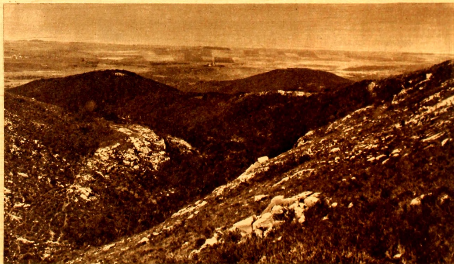
FORMAS MENORES QUE LA EROSION TIENDE A SEPARAR LENTAMENTE DE LA PORCION MERIDIONAL DEL CERRO DE LAS ANIMAS, MALDONADO.
