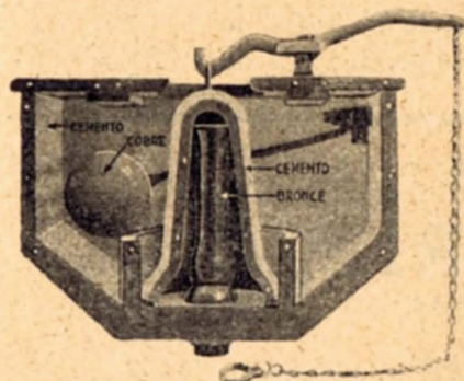
SECCION LONGITUDINAL
