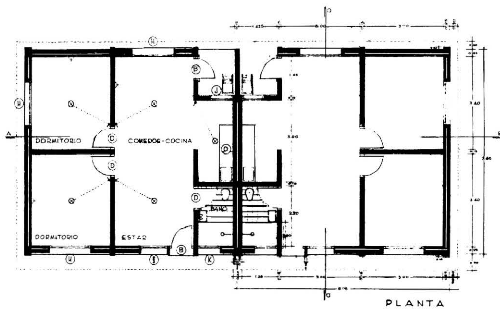
Vivienda Tipo "P2a"
