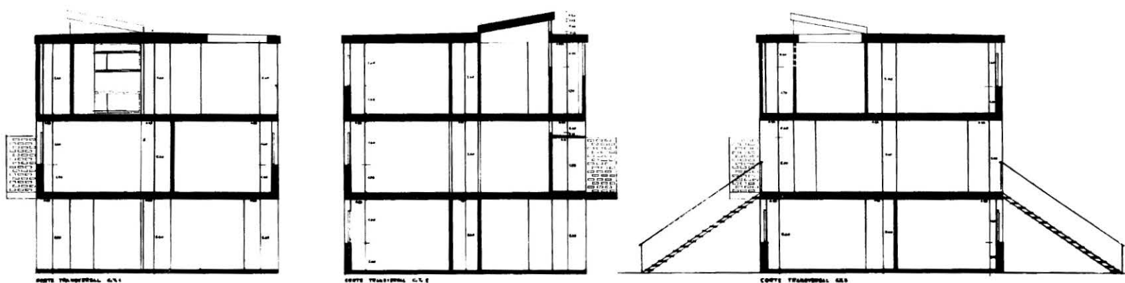
Unidad tipo "U 1" - Cortes
