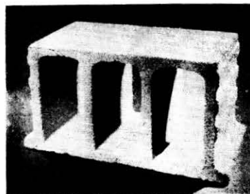
BOVEDILLAS Tipo 25 50 × 25 × 25 2 Apoyos
