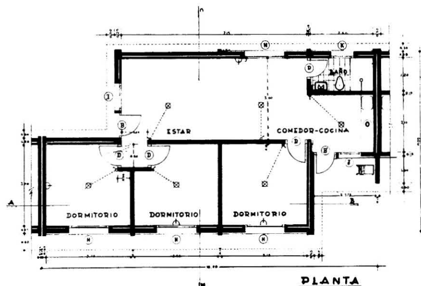
Vivienda Tipo "S3b" - Barrio B2 - Maldonado
