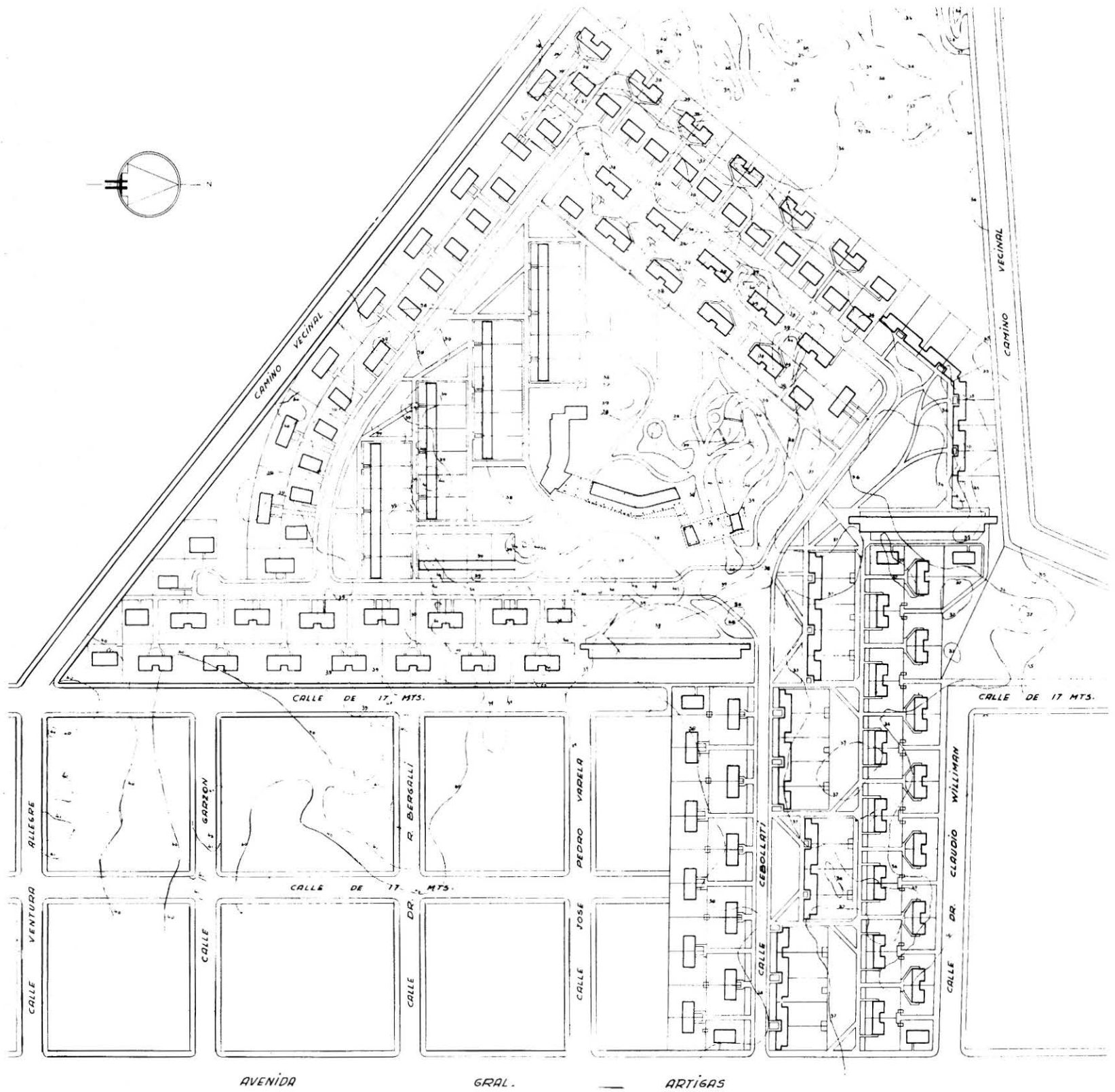
Planta de Ubicación - Barrio B-2 - Maldonado
