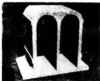
BOVEDILLAS Tipo 35 25 × 40 × 35 2 Apoyos
