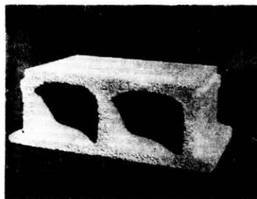
BOVEDILLAS Tipo 15 25 × 40 × 15 2 Apoyos
