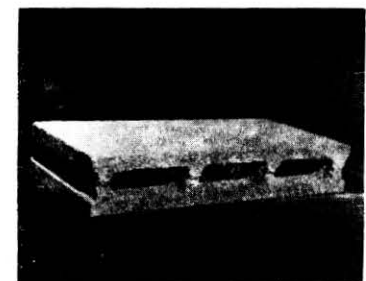
BLOQUES Tipo 7 7 × 20 × 40
