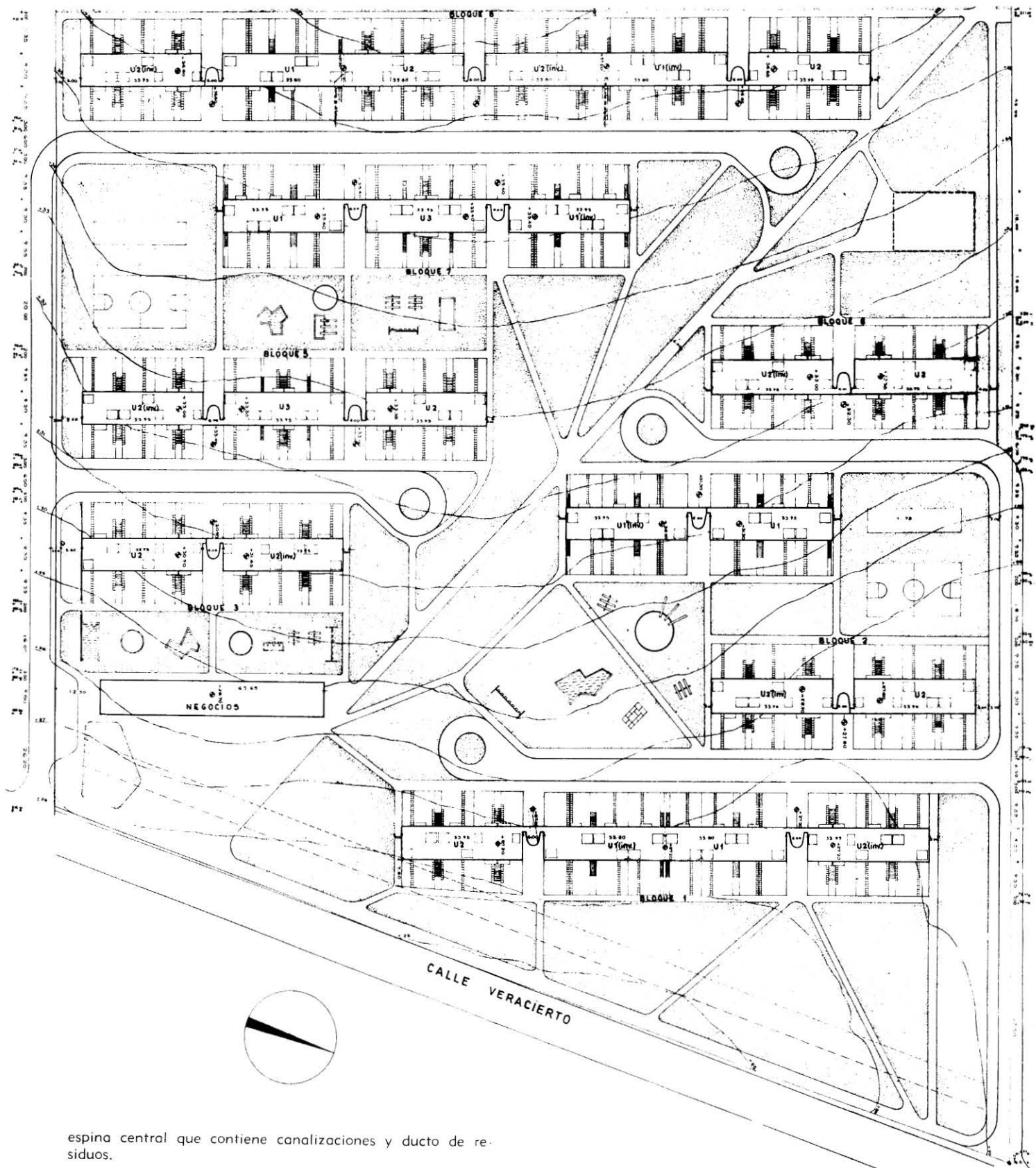
Planta de Ubicación - Barrio N° 16 - Montevideo
