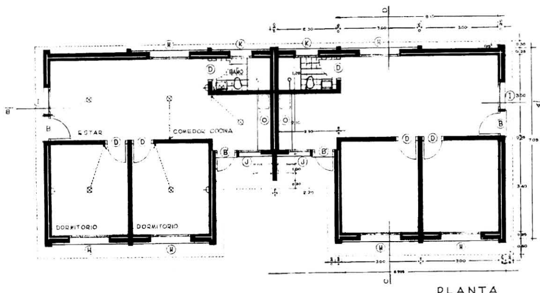
Vivienda Tipo "P2b" - Barrio B-2 - Maldonado
