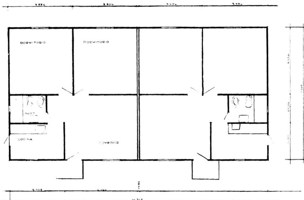
Vivienda Tipo "A" Barrios Nos. 14 y 15
