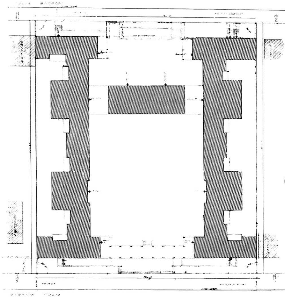
Planta de Ubicación - Casa Colectiva Nº 1 - Montevideo
