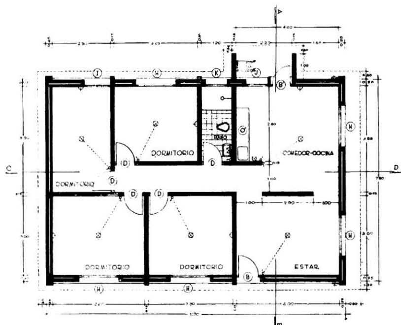
Vivienda Tipo "U4a" - Barrio B-2 - Maldonado
