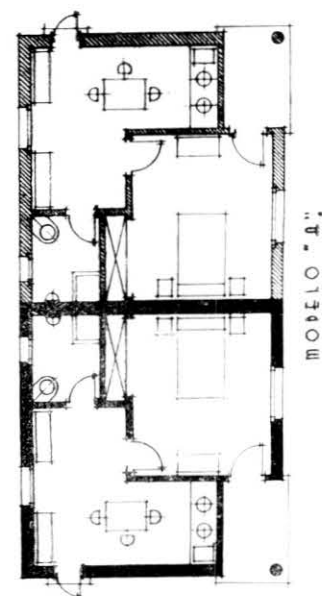
PLANTA DEL MODELO A
