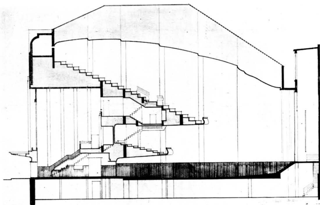
CORTE LONGITUDINAL DE LA SALA
