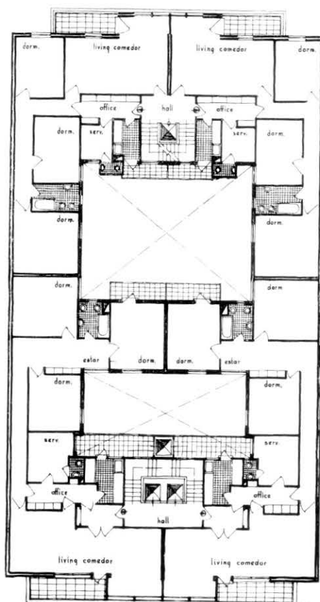
PLANTA TIPO 1º A 5º PISO.
