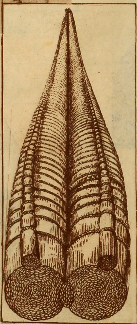
Corte de una balsa, ejecutado se- gún el ejemplar del Museo Nacio- nal de Historia Natural.
