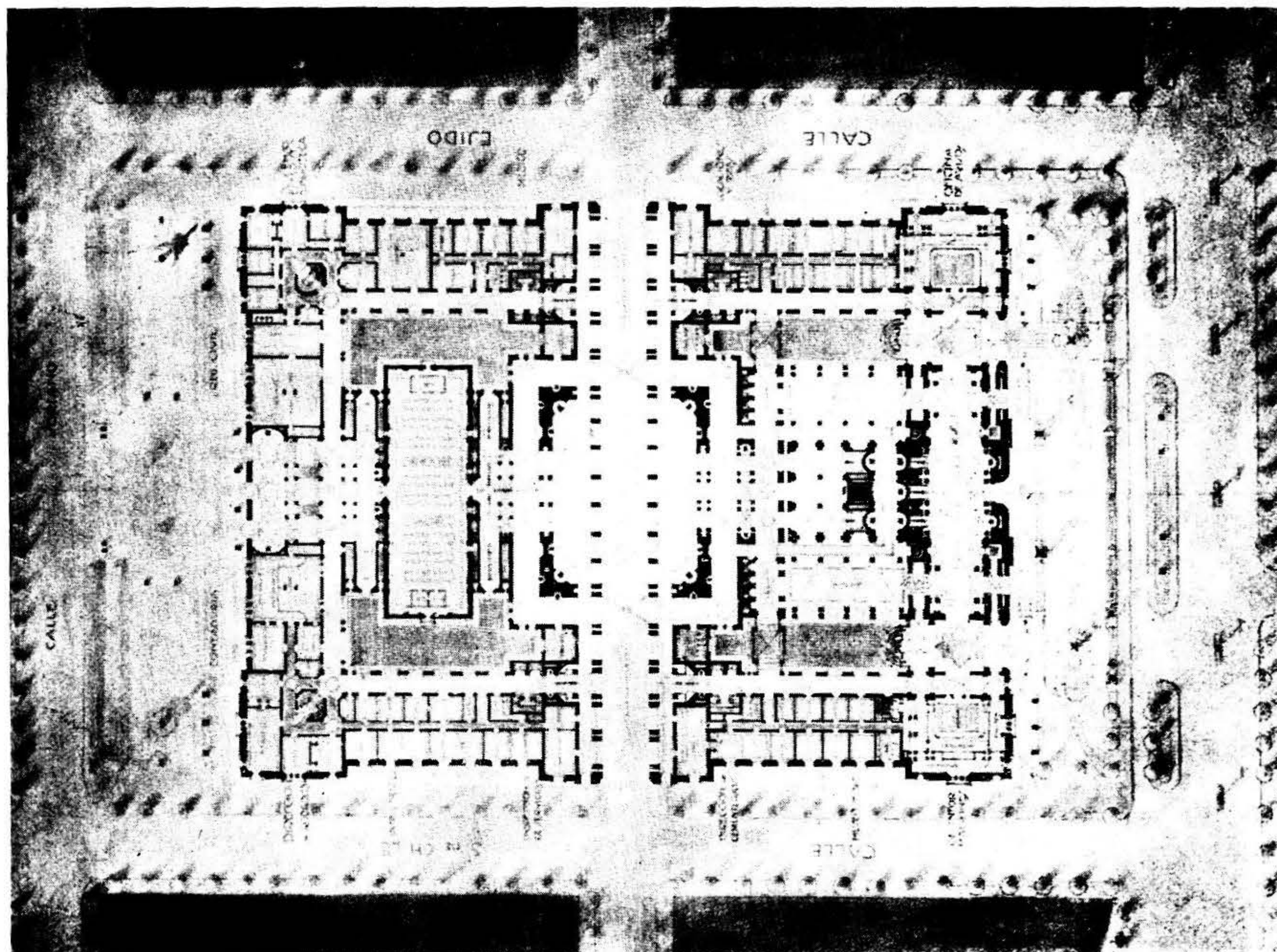
PLANTA DEL BASAMENTO
