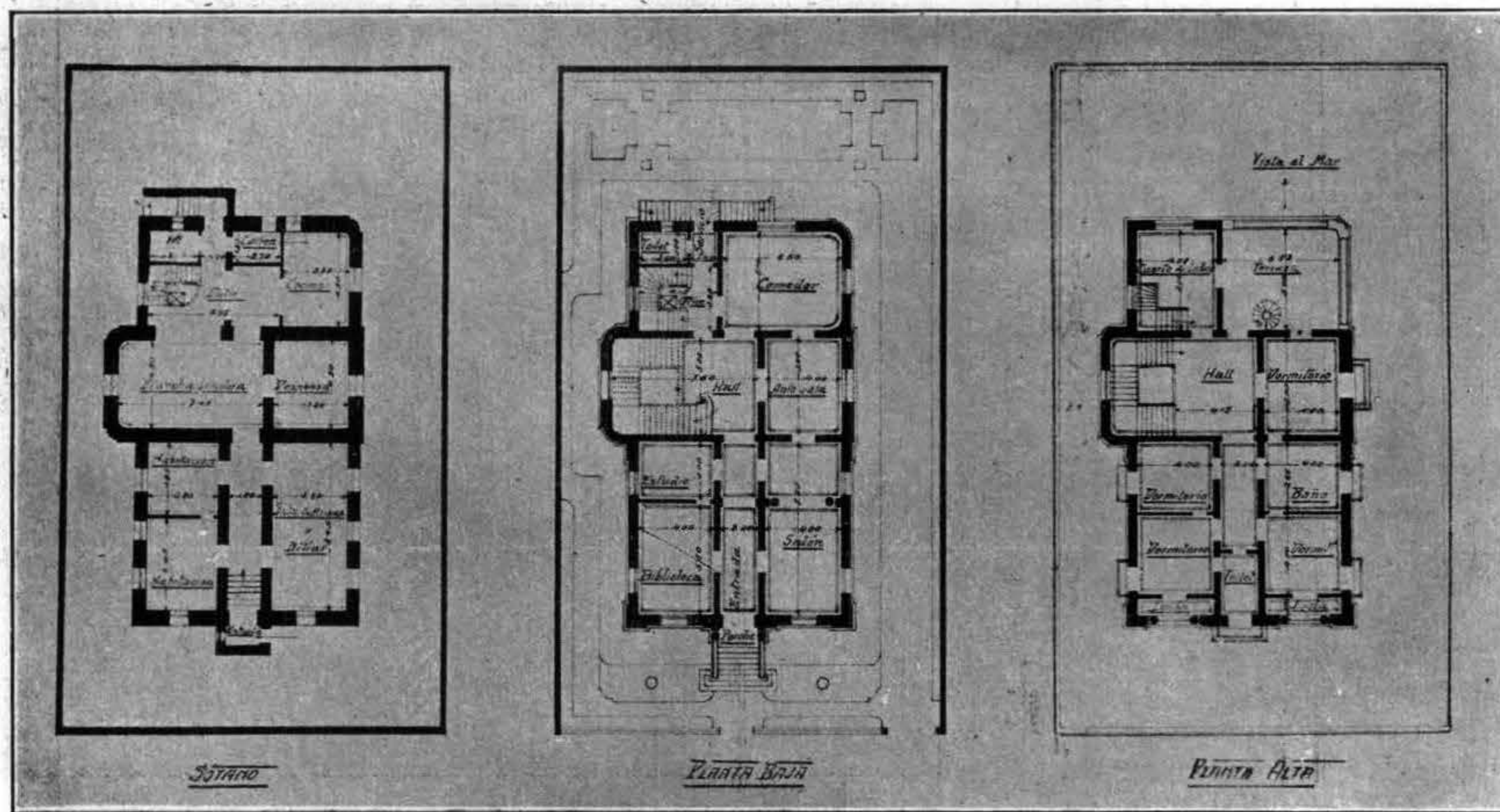
ARQ. ALFREDO R. CAMPOS. — UN HOTEL PARTICULAR
