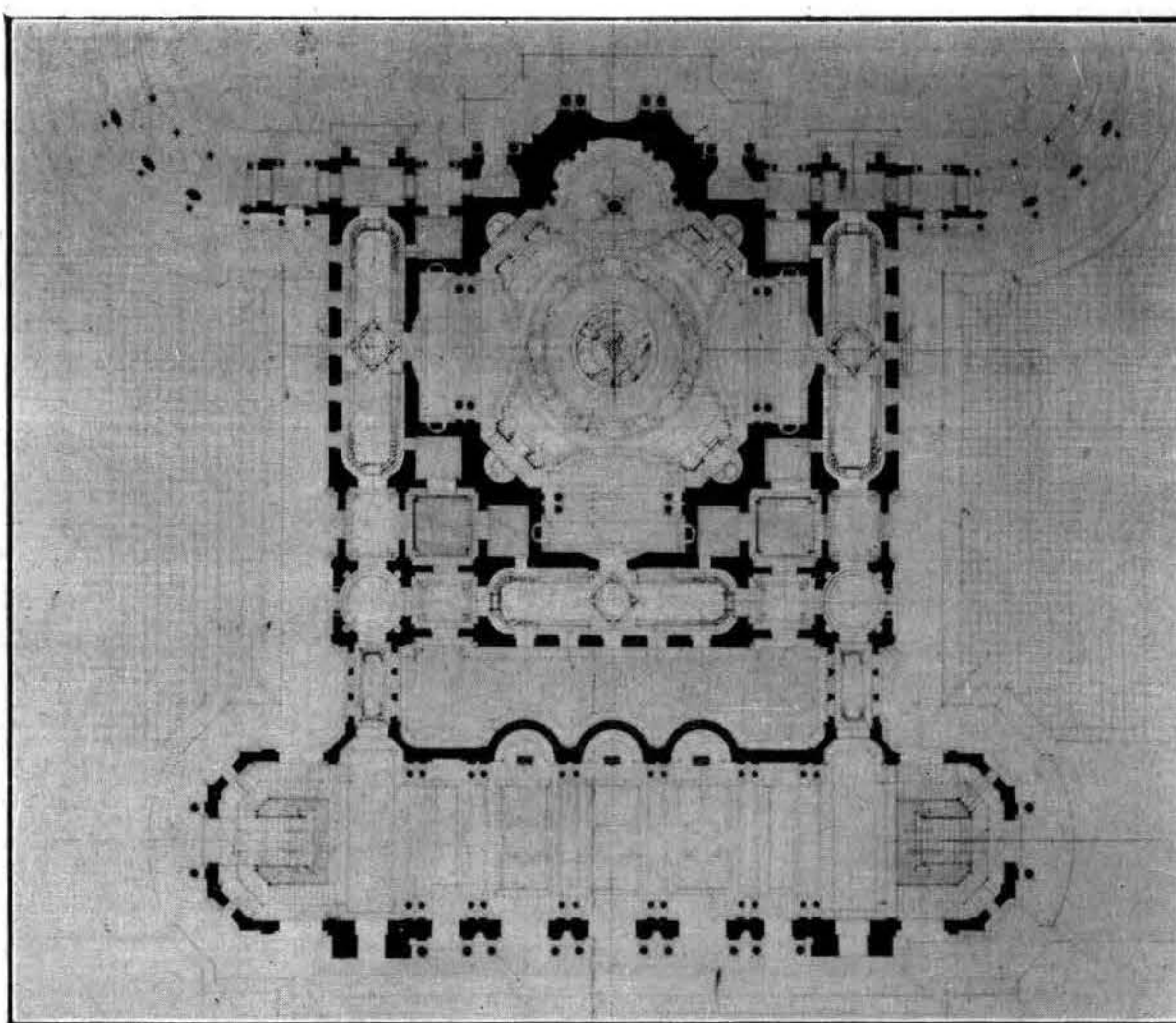
G. RODRÍGUEZ LARRETA. — UN SALÓN DE LA PAZ. — PROYECTO DE COMPOSICIÓN DECORATIVA
