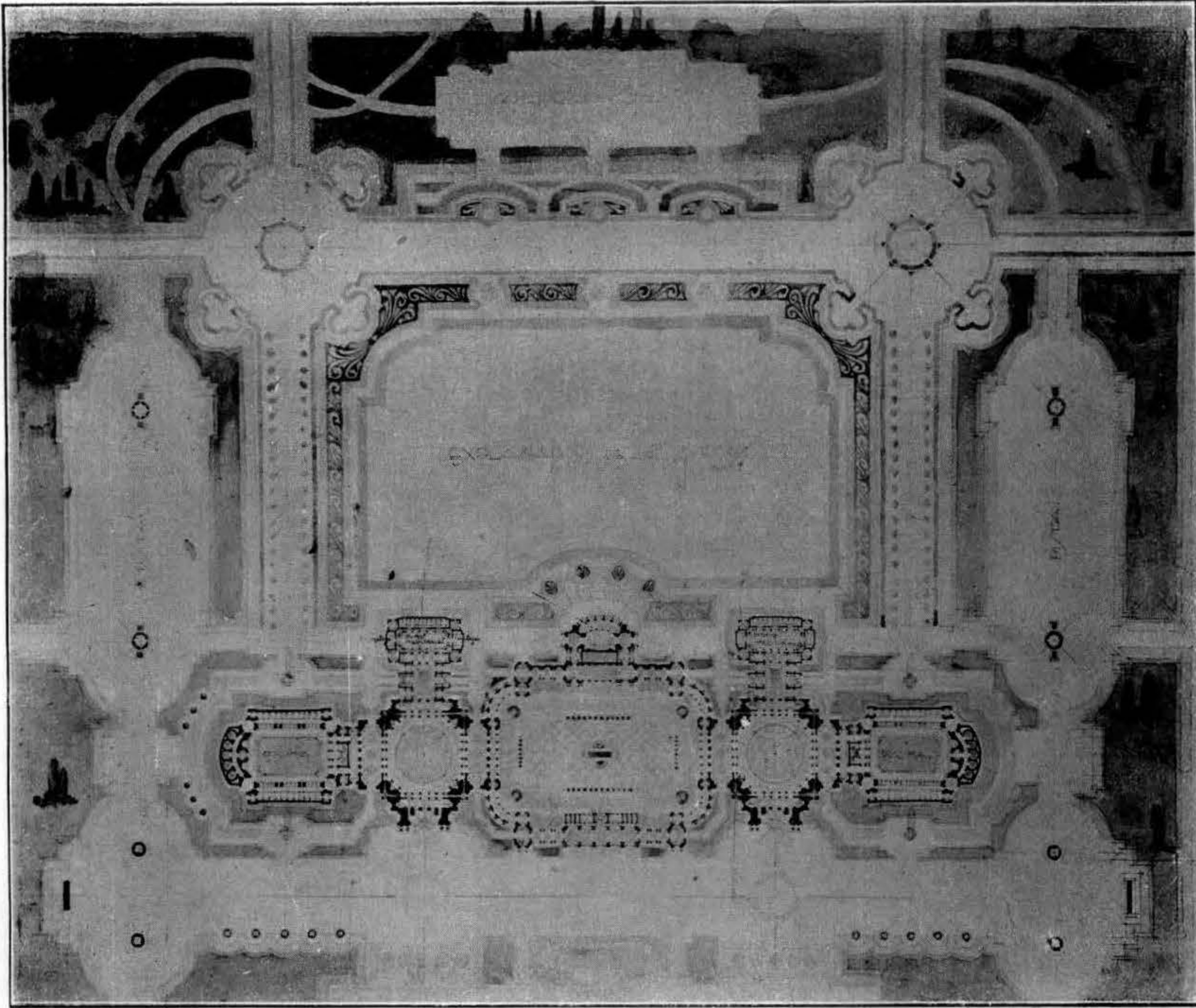
JULIO VILAMAJÓ.—UN ESTABLECIMIENTO DE BAÑOS.—CONCURSO DE ARQUITECTURA 4.º CURSO
