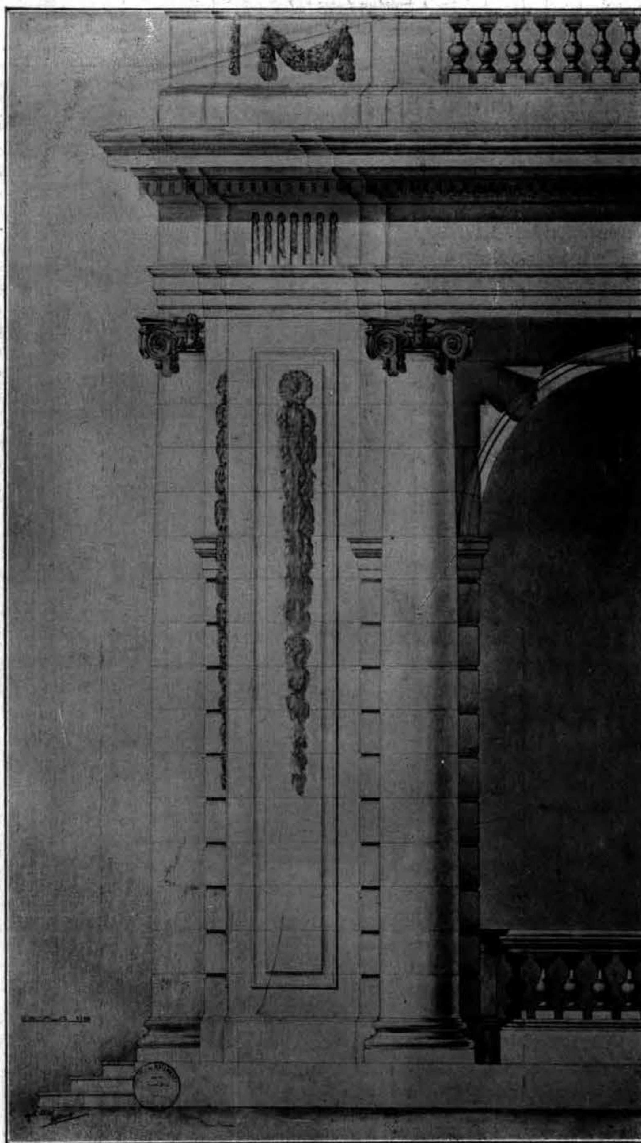
R. CAPRARIO. — PROYECTO DE ÓRDENES DE ARQUITECTURA
