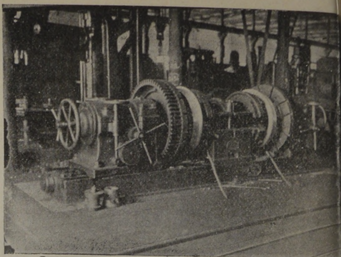
Operación de montaje.—Torno para la fabricación de las yantas de las ruedas de vagones
