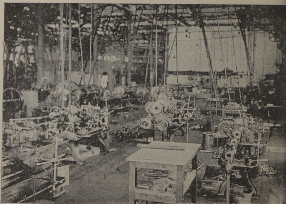
Máquinas pulidoras
