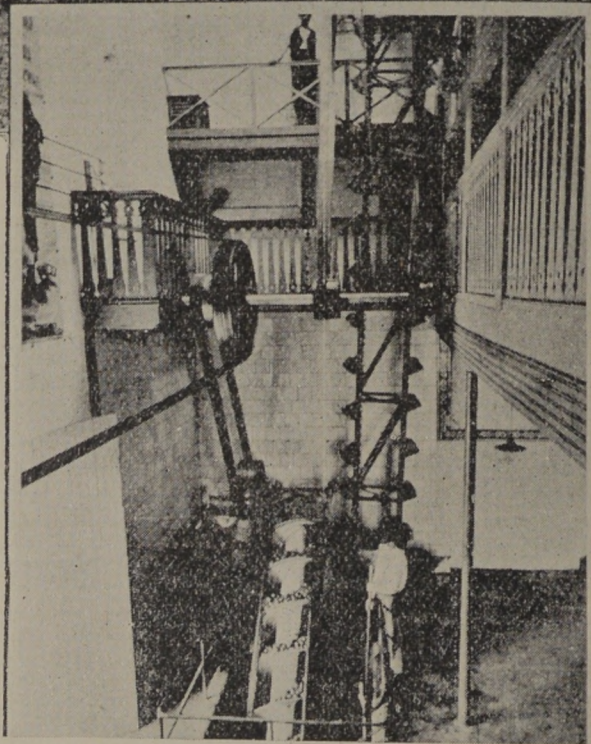
Elevador de manzana, movido por fuerza eléctrica, en que aparece el tornillo sin fin y los cangilones armados.
