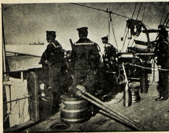
Pieza Armstrong de 152 y piezas de desembarco.
