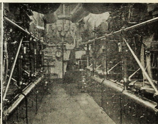
Estación telegráfica (tel. sin hilo).—Salón de máquinas
