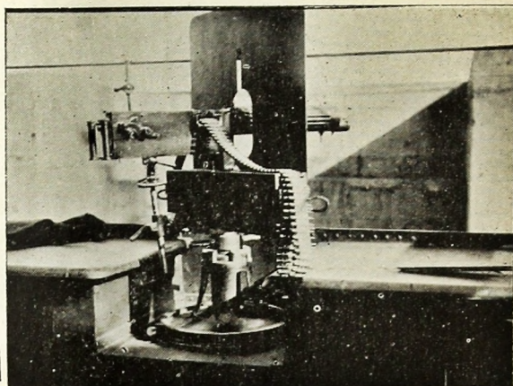
Tubo lanza torpedo Whitehead, mostrando el torpedo.— Ametralladora Vicker-Maxin
