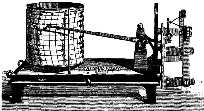
Higrógrafo Richard
