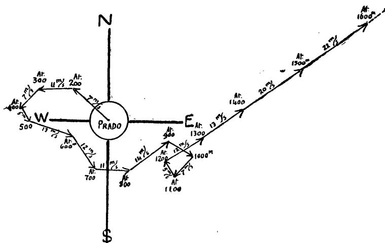
Trayectoria de un globo piloto
